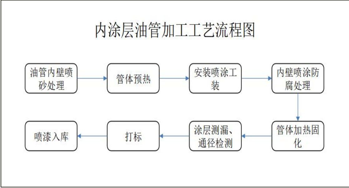
图4-1 内涂层油管产品生产工艺流程图
