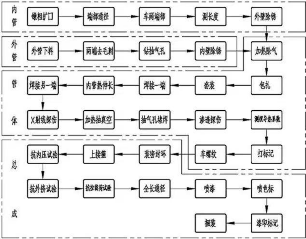
图4-1 隔热油管生产工艺流程图
